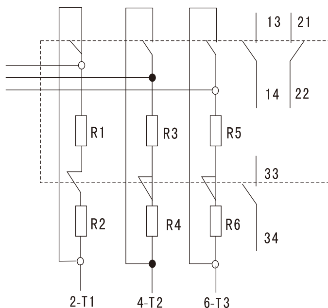
CJ19(16B)-63\95电路原理图
