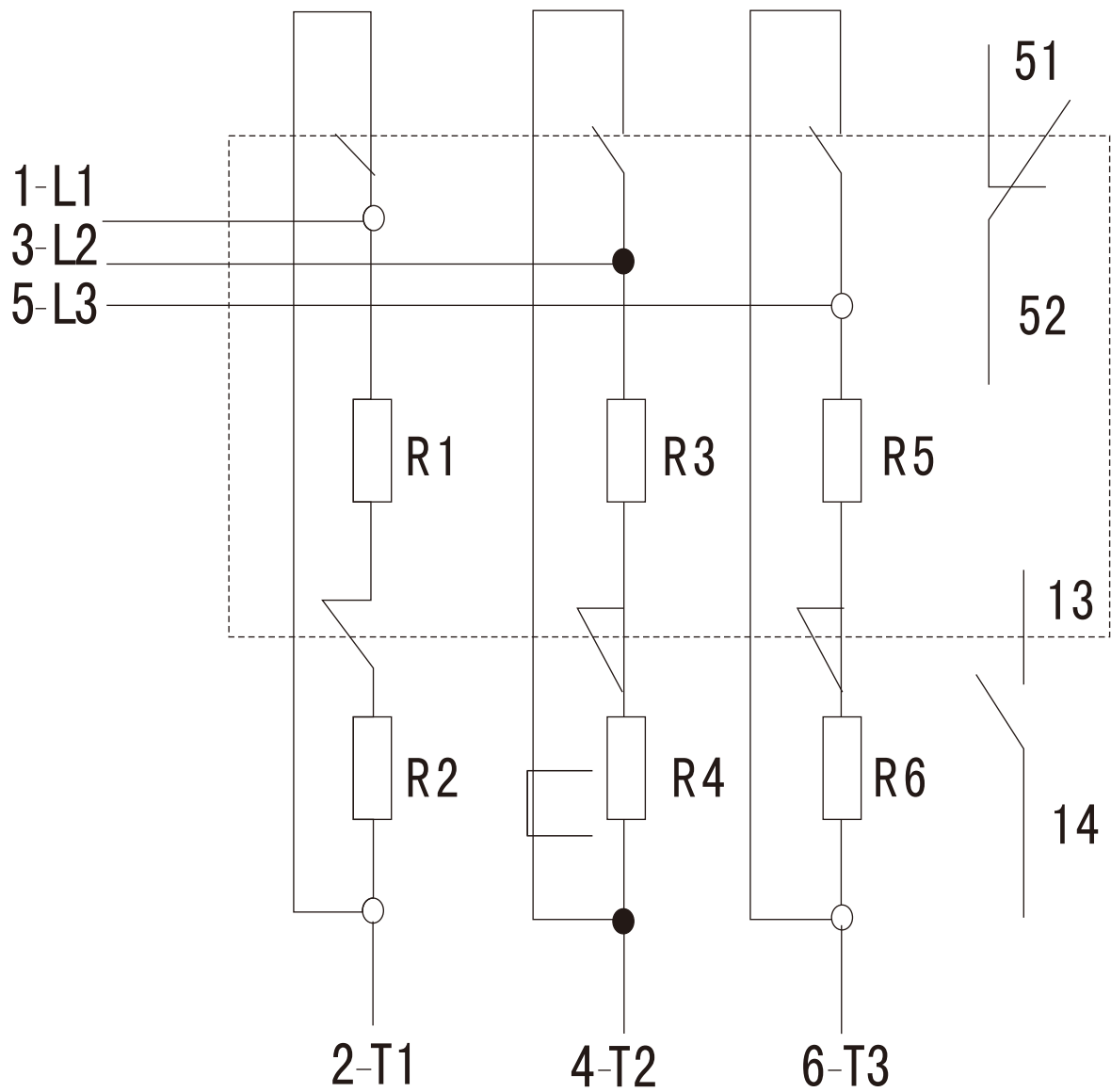
CJ19 (16B)-25、43\11 电路原理图
