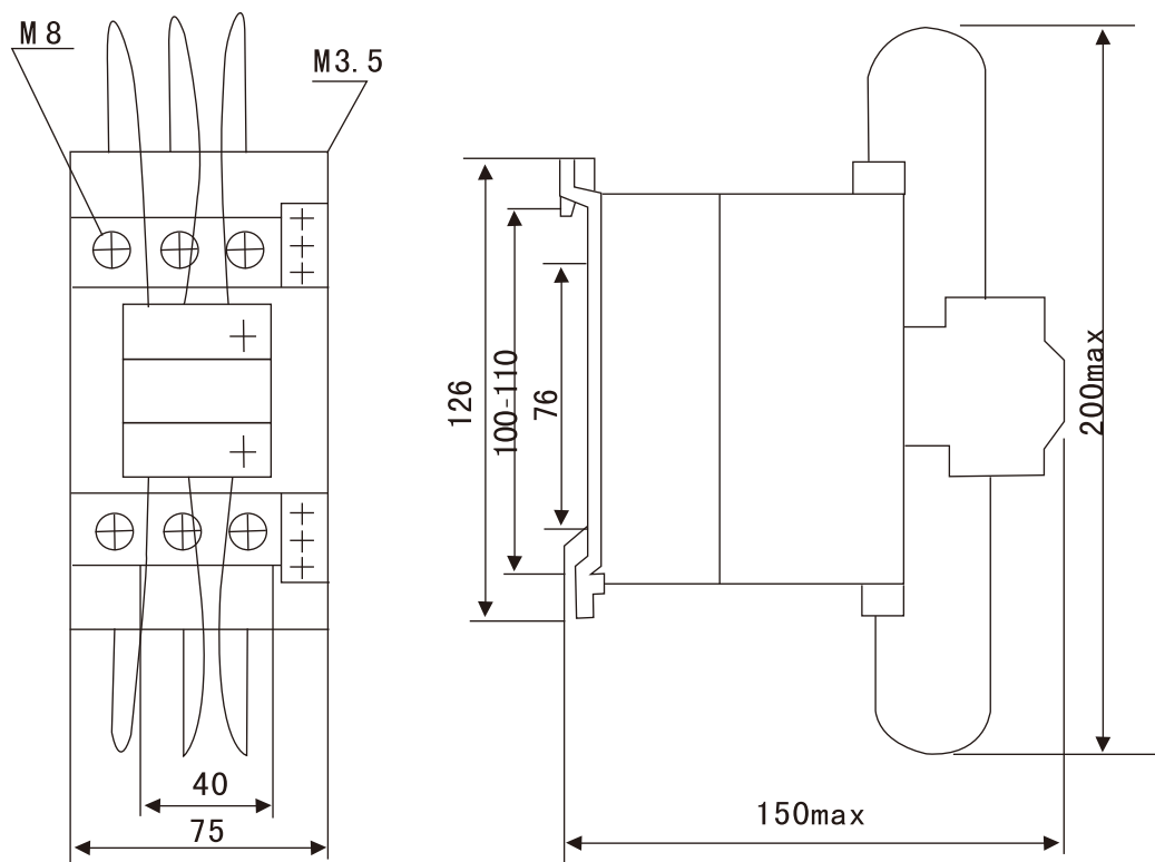
CJ19(16B)-63、95外形尺寸及安装尺寸
