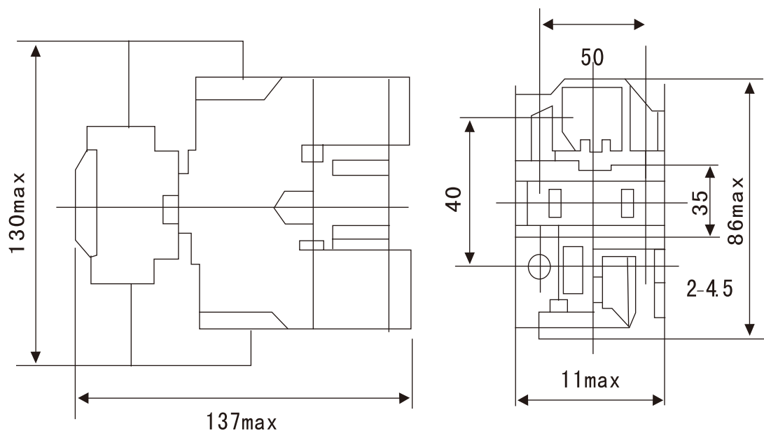
CJ19 (16B)-25、32、43 外形尺寸及安装尺寸
